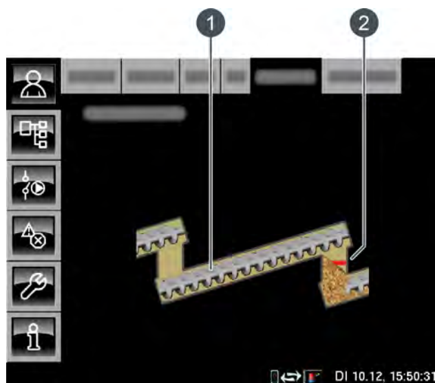
Fig. 8-34: Aperçu Vis sans fin intermédiaire
