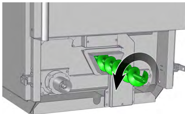
Fig. 10-4: Dévisser la vis de décendrage
