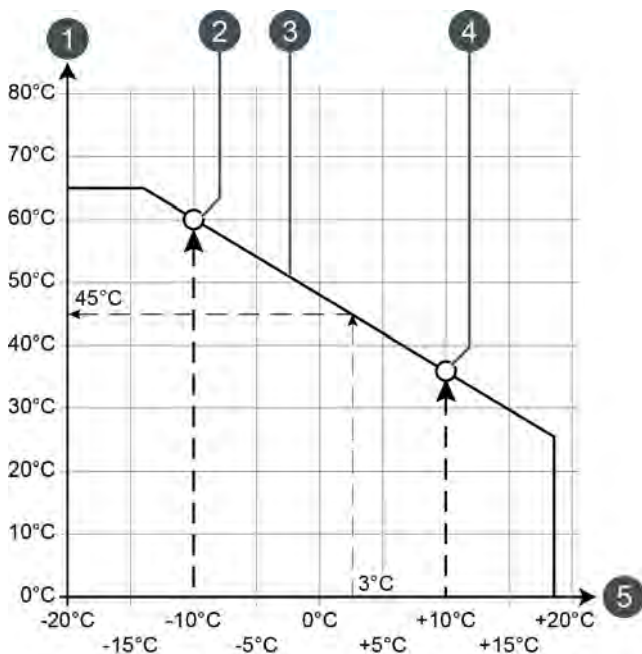
Fig. 8-18: Courbe de chauffage [Jour]
