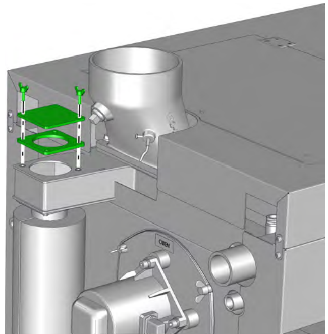
Fig. 7-2: Dépose de la trappe de visite
