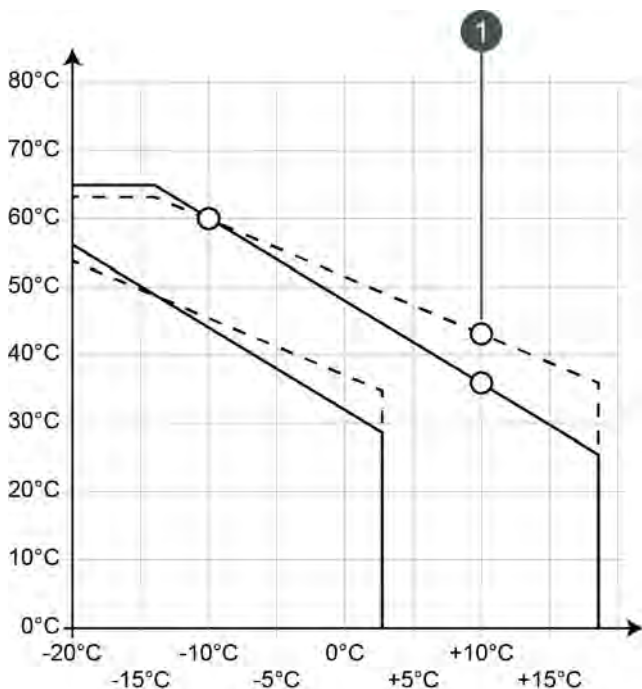
Fig. 8-20: Adapter la courbe de chauffage au cours de la période de transition
