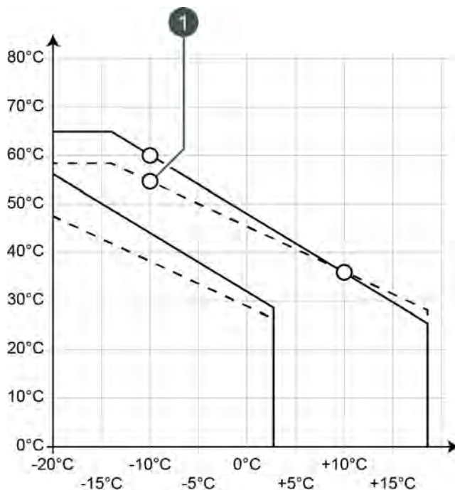
Fig. 8-21: Adapter la courbe de chauffage en hiver
