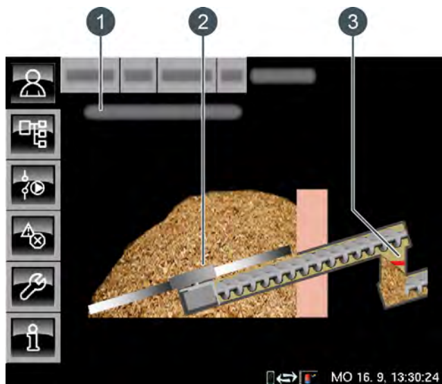
Fig. 8-36: Aperçu Extraction externe
