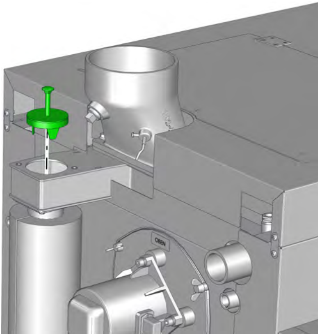
Fig. 7-3: Couvercle d'arrêt
