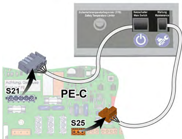
Fig. 10-15: Débrancher les câbles de l'alimentation réseau et de l'interrupteur de maintenance
