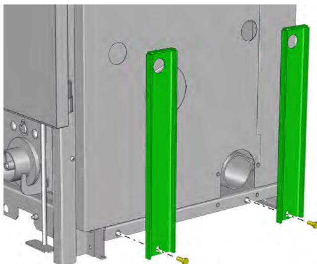
Fig. 10-1: Plaques de traction
