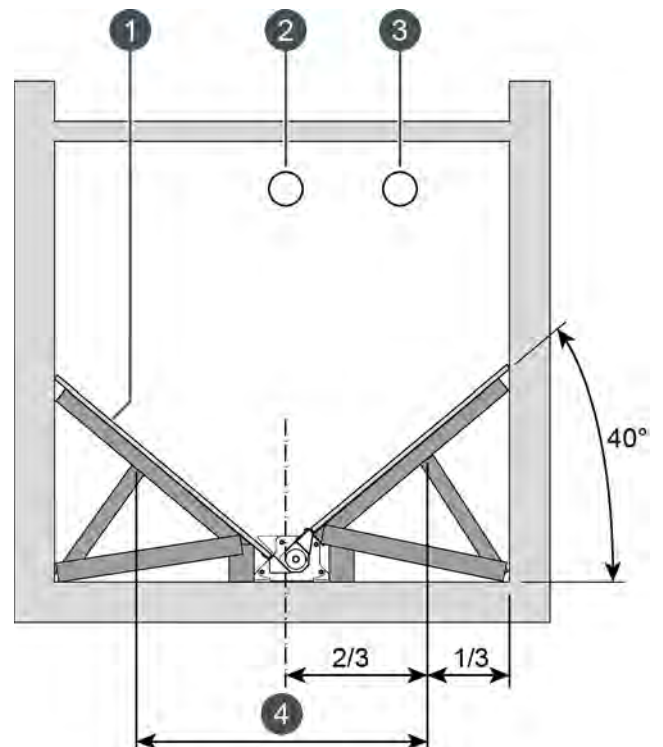
Fig. 13-7: Construction du plancher incliné pour la vis d'alimentation
