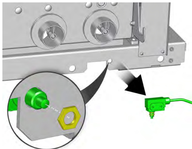
Fig. 10-25: Capteur de position du cendrier
