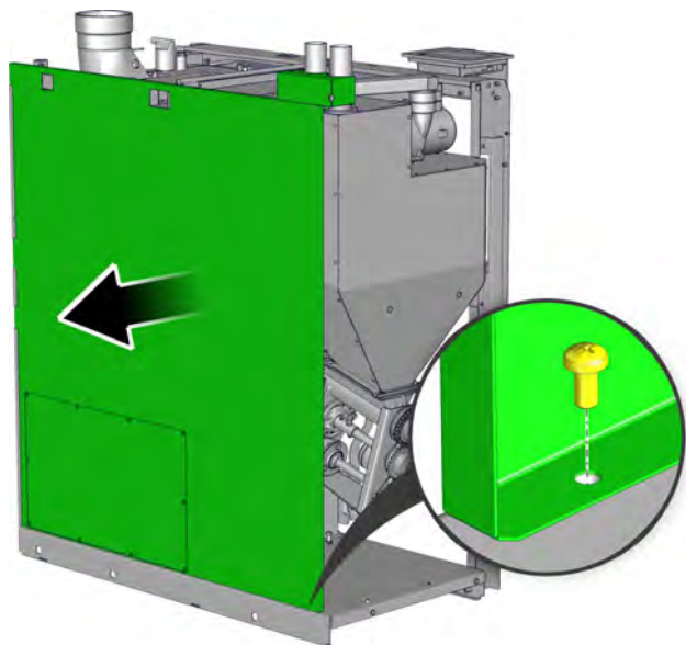
Fig. 10-12: Revêtement
