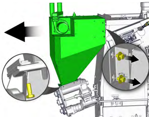
Fig. 10-22: Réservoir
