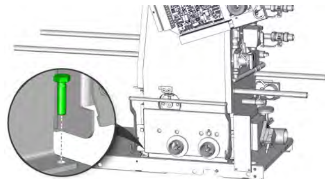
Fig. 10-26: Desserrer les vis
