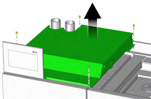
Fig. 10-10: Revêtement
