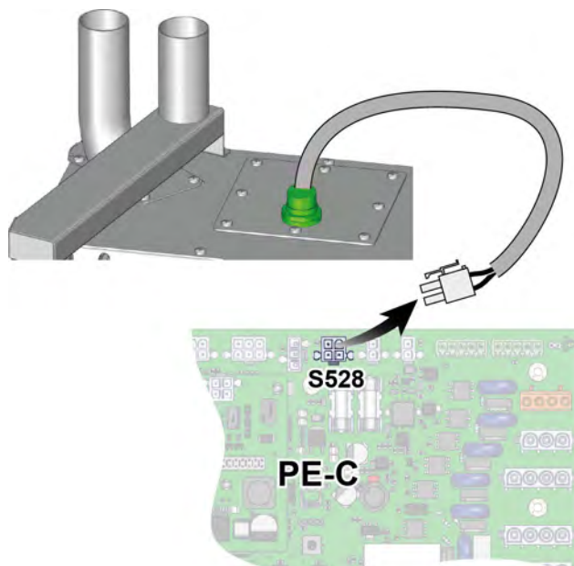
Fig. 10-21: Capteur de niveau de remplissage
