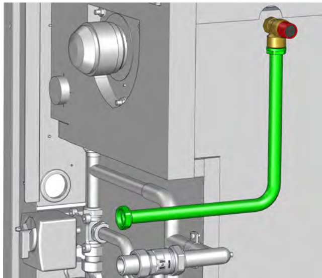
Fig. 10-28: Soupape de sécurité de la chaudière
