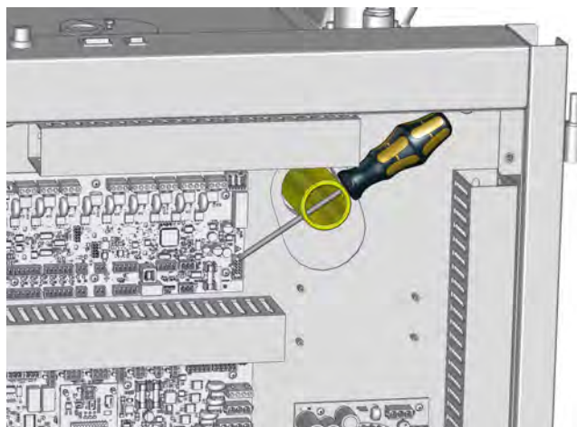
Fig. 10-17: Fixer le support de platine
