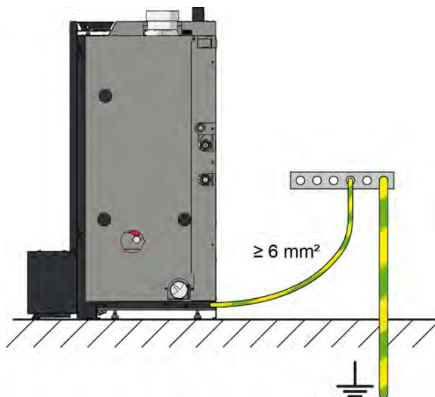
Fig. 10-30: Raccorder la liaison équipotentielle
