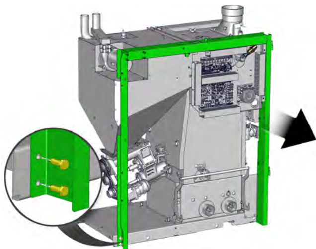
Fig. 10-18: Cadre
