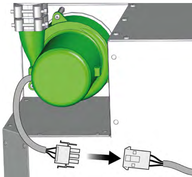
Fig. 10-20: Turbine d'aspiration
