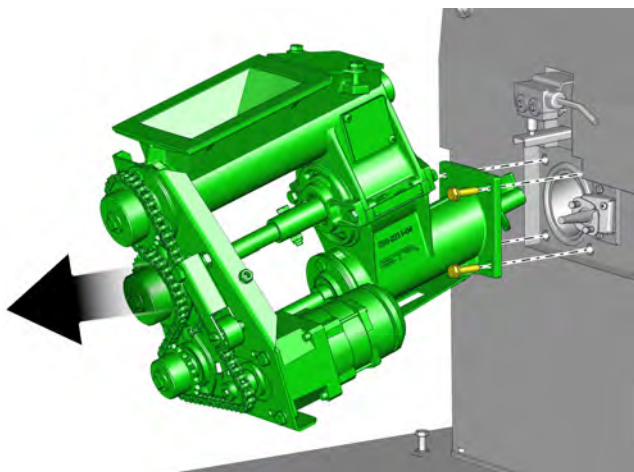
Fig. 10-23: Vis d'alimentation
