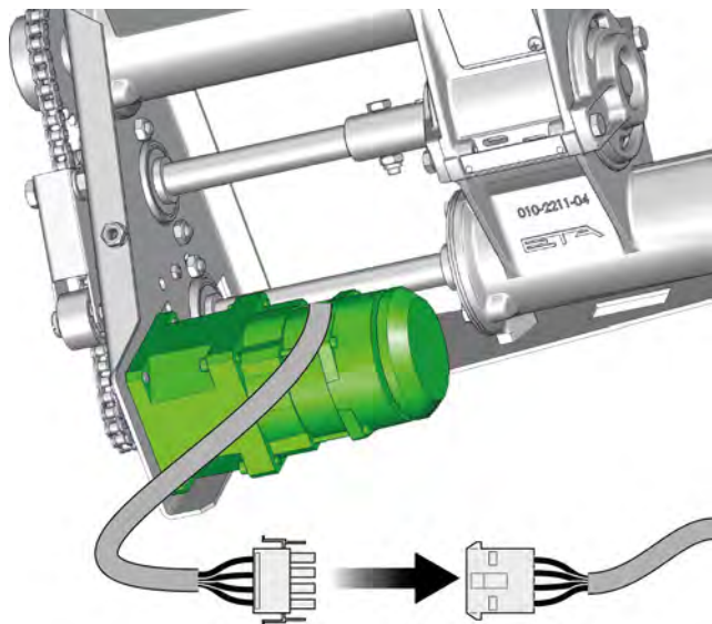
Fig. 10-19: Entraînement de la vis d'alimentation
