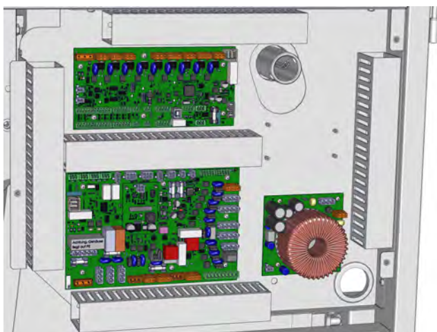
Fig. 10-8: Platines
