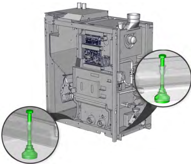
Fig. 10-27: Pieds articulés
