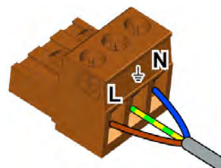
Fig. 11-1: Ligne d'alimentation
