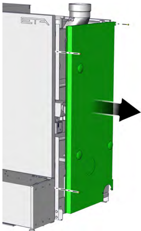
Fig. 10-5: Revêtement latéral
