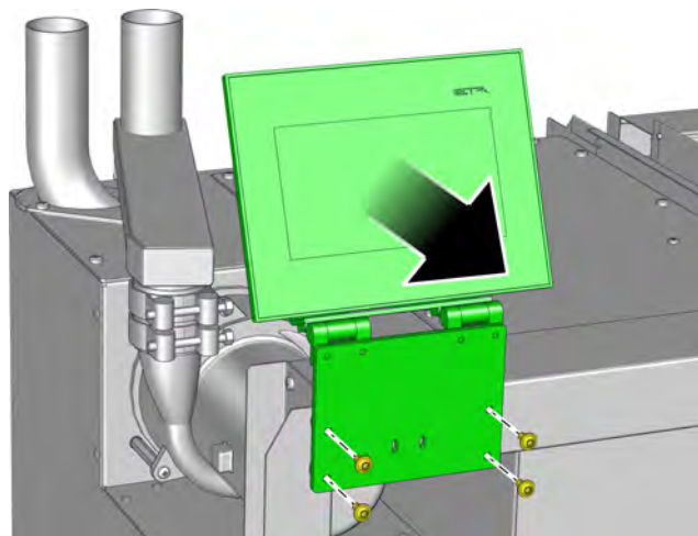
Fig. 10-14: Retirer l'écran
