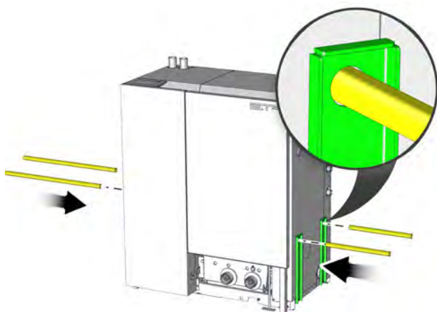
Fig. 10-2: Barres de levage
