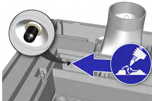
Fig. 2-23: Tête de la sonde lambda
