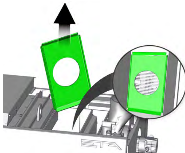
Fig. 2-38: Couvercle de la chambre de combustion
