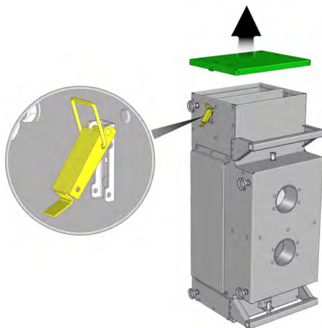
Fig. 2-6: Couvercle
