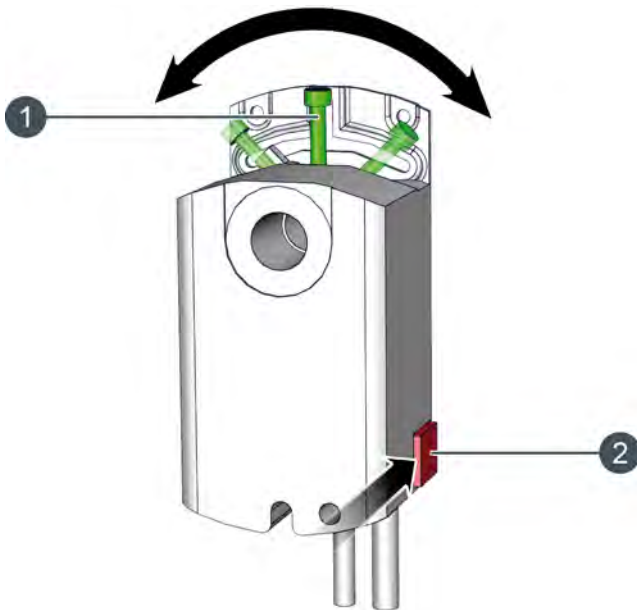
Fig. 2-62: Actionner manuellement le moteur de réglage
