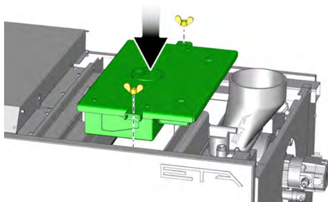
Fig. 2-26: Couvercle de l'échangeur de chaleur
