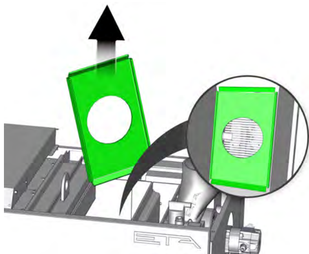
Fig. 2-18: Couvercle de la chambre de combustion
