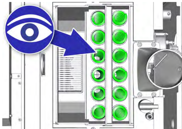
Fig. 2-42: Tubes de l'échangeur de chaleur
