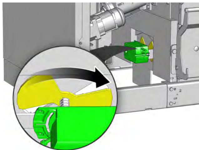
Fig. 2-61: Moteur de réglage de l'air secondaire
