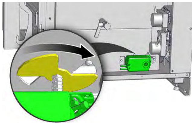
Fig. 2-60: Moteur de réglage de l'air primaire
