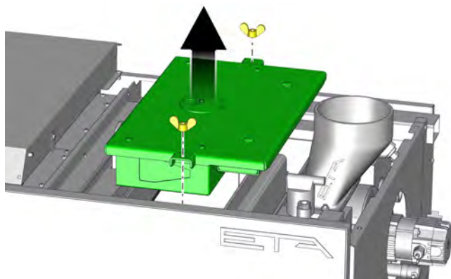
Fig. 2-37: Couvercle de l'échangeur de chaleur
