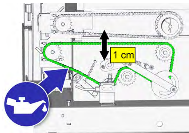
Fig. 2-59: Chaîne d'entraînement de l'évacuation des cendres
