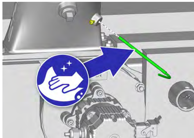
Fig. 2-35: Sonde de température des fumées
