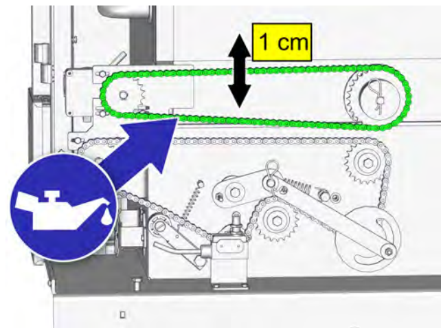
Fig. 2-58: Chaîne d'entraînement de la grille
