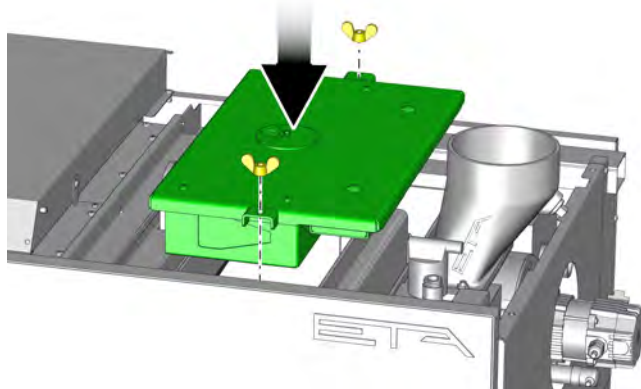
Fig. 2-44: Couvercle de l'échangeur de chaleur
