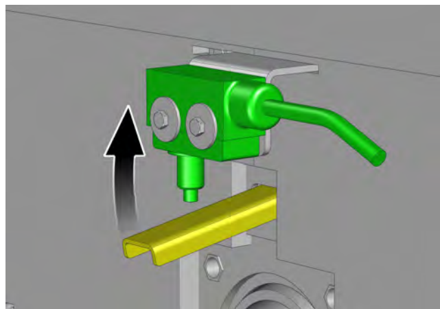
Fig. 2-40: Interrupteur du lit de braises
