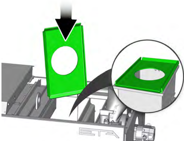
Fig. 2-22: Couvercle de la chambre de combustion
