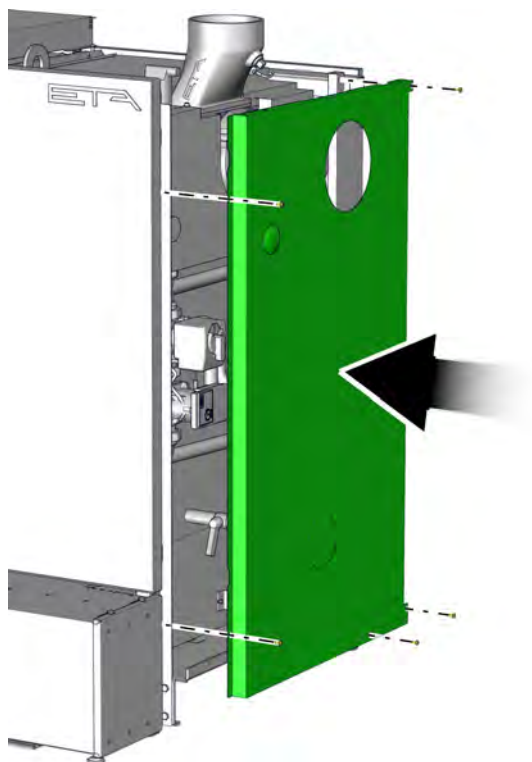
Fig. 2-64: Revêtement latéral
