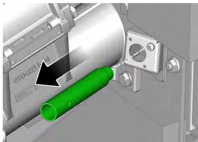
Fig. 2-48: Tube d'allumage
