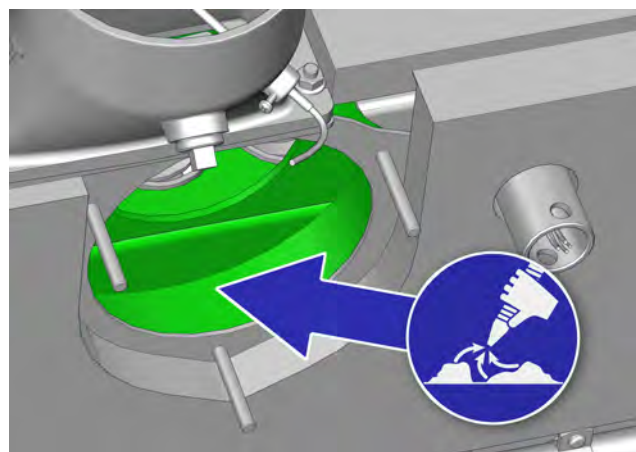
Fig. 2-33: Nettoyer le logement du ventilateur
