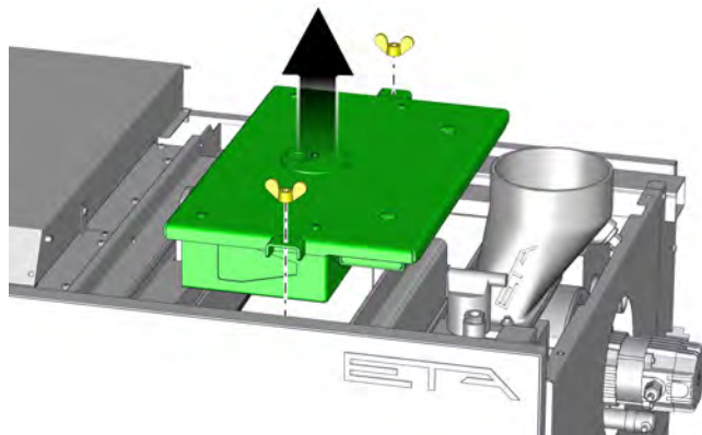
Fig. 2-17: Couvercle de l'échangeur de chaleur
