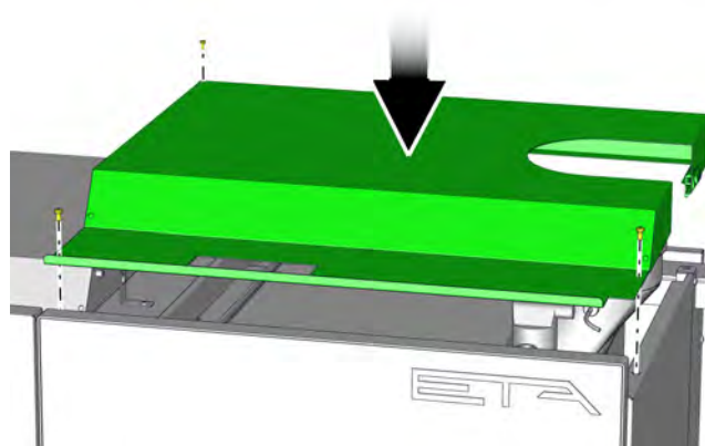
Fig. 2-28: Revêtement
