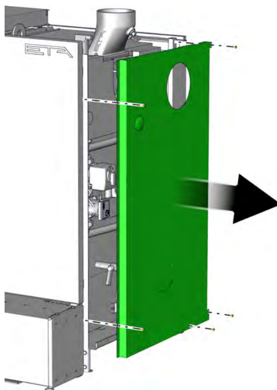
Fig. 2-30: Revêtement latéral
