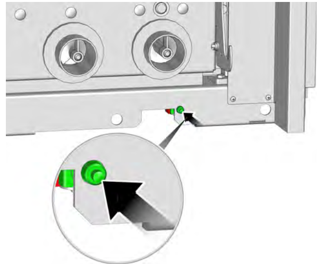
Fig. 2-63: Capteur de position du cendrier
