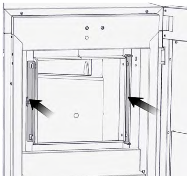
Fig. 7-11: Déplacer la charnière et le support du rouleau de fermeture
