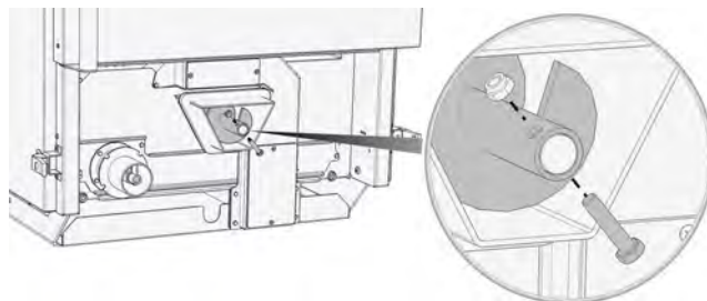
Fig. 11-3: Enlever la vis
