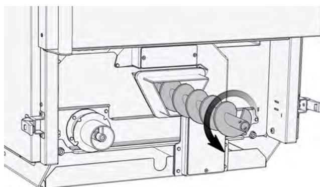
Fig. 11-4: Dévisser la vis de décendrage
