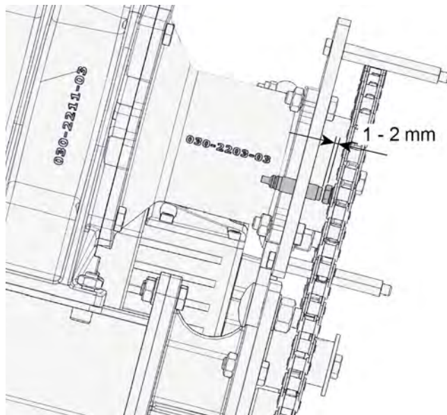
Fig. 7-15: Écart entre le capteur et la vis
