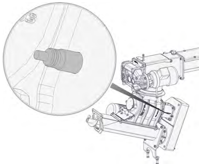
Fig. 7-14: Capteur de position du sas rotatif
