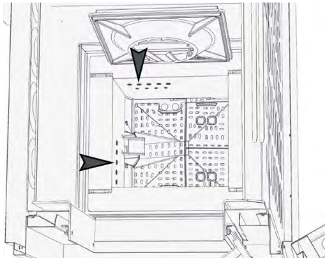
Fig. 7-3: Orifices d'air secondaire
