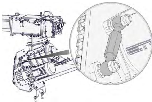
Fig. 7-5: Tendeur
