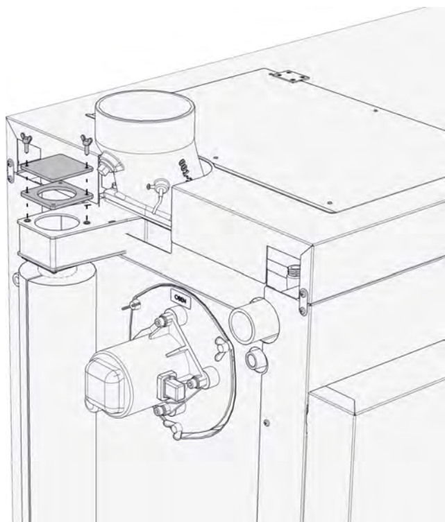
Fig. 8-3: Retirer la trappe de visite
