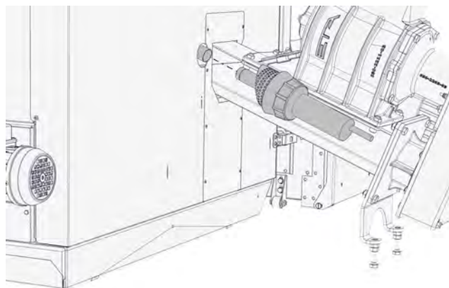
Fig. 7-12: Retirer l'allumeur
