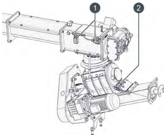
Fig. 7-13: Interrupteur de sécurité
