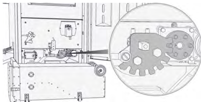
Fig. 7-9: Entraînement de fuseau et engrenage
