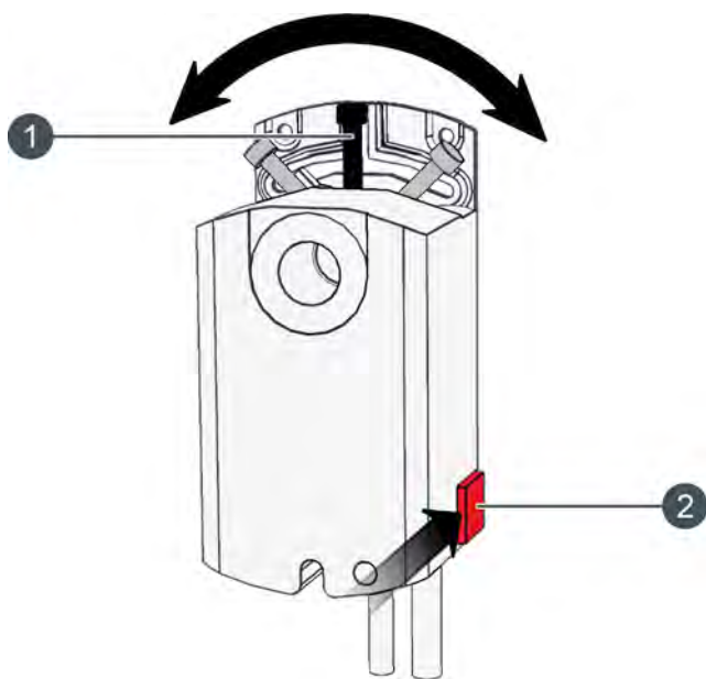
Fig. 7-8: Actionner manuellement le moteur de réglage
