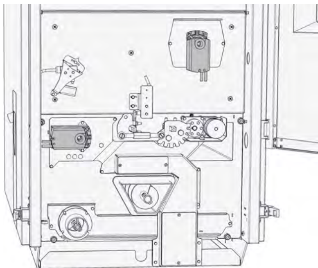
Fig. 7-7: Moteurs de réglage pour les valves d'air
