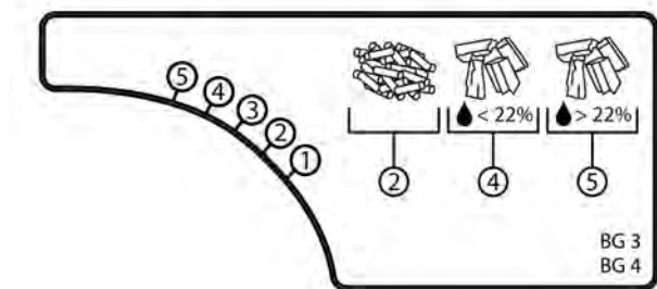
Fig. 8-2: Positions du capteur de niveau du lit de braises
