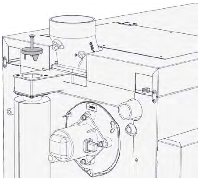
Fig. 8-4: Couvercle d'arrêt
